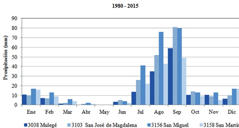
Figura 4. Precipitación promedio mensual en la región de la cuenca de Mulegé, para el periodo de 1980 al 2015 (SMN, 2009; CLICOM, 2015).
